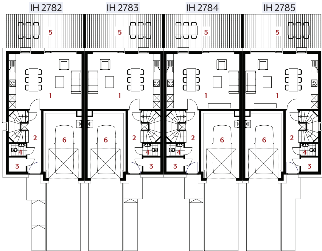
REZ-DE-CHAUSSEE
